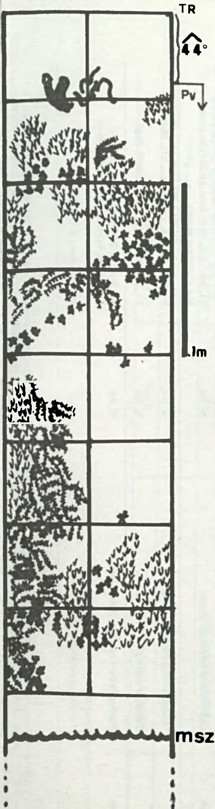
Fig. 7 - Transect na face sul da rocha (fig. 4a), desde o topo (TR) até o nível de maré alta de sizígia (msz), ao longo de um paredão vertical (Pv). Símbolos: Brassavola tuberculata [V V V]; Cephalocereus fluminensis [C]; Polypodium lanceolatum [P]; Selenicereus setaceus [S]; Tillandsia stricta [T]
