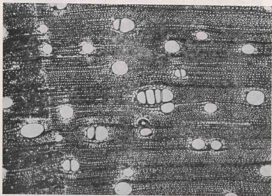
Plathymentia reticulata Benth. (amostra n.º 3010-SBG) Foto 14 — Secção transversal do cerne (x 50)
