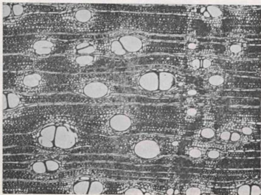
Plathymentia foliolosa Benth. (amostra n.º 3009-SBG) Foto 13 — Secção transversal (x 50)
