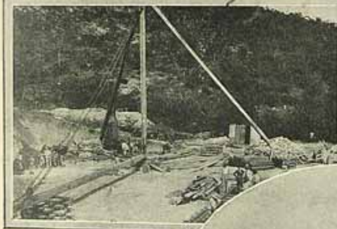
Açude de Piranhas. Escriptorio dos technicos encarregados da construção. Trabalhos preparatorios. Construção da torre para o cabo aereo destinado a transportar os pesados blocos de concreto que formarão a barragem.
