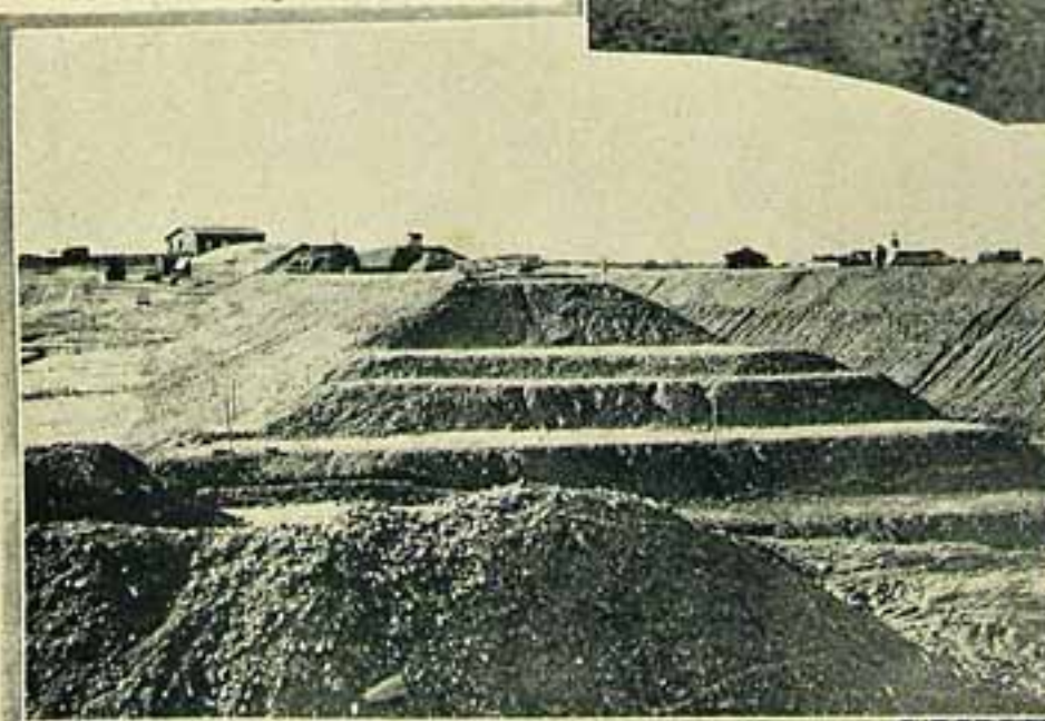
ESTADO DA PARAÍBIA DO NORTE: BARRAGEM DE TERRA EM CONSTRUÇÃO. PONTE DE CIMENTO ARMADO EM CONSTRUÇÃO SOBRE O RIO PARAÍBIA, EM ITABAYANA.
