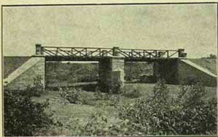
Ponte Bôa-Vista, na Estrada de Rodagem Bôa-Vista a Ca- becciras — Kilometro 19.
