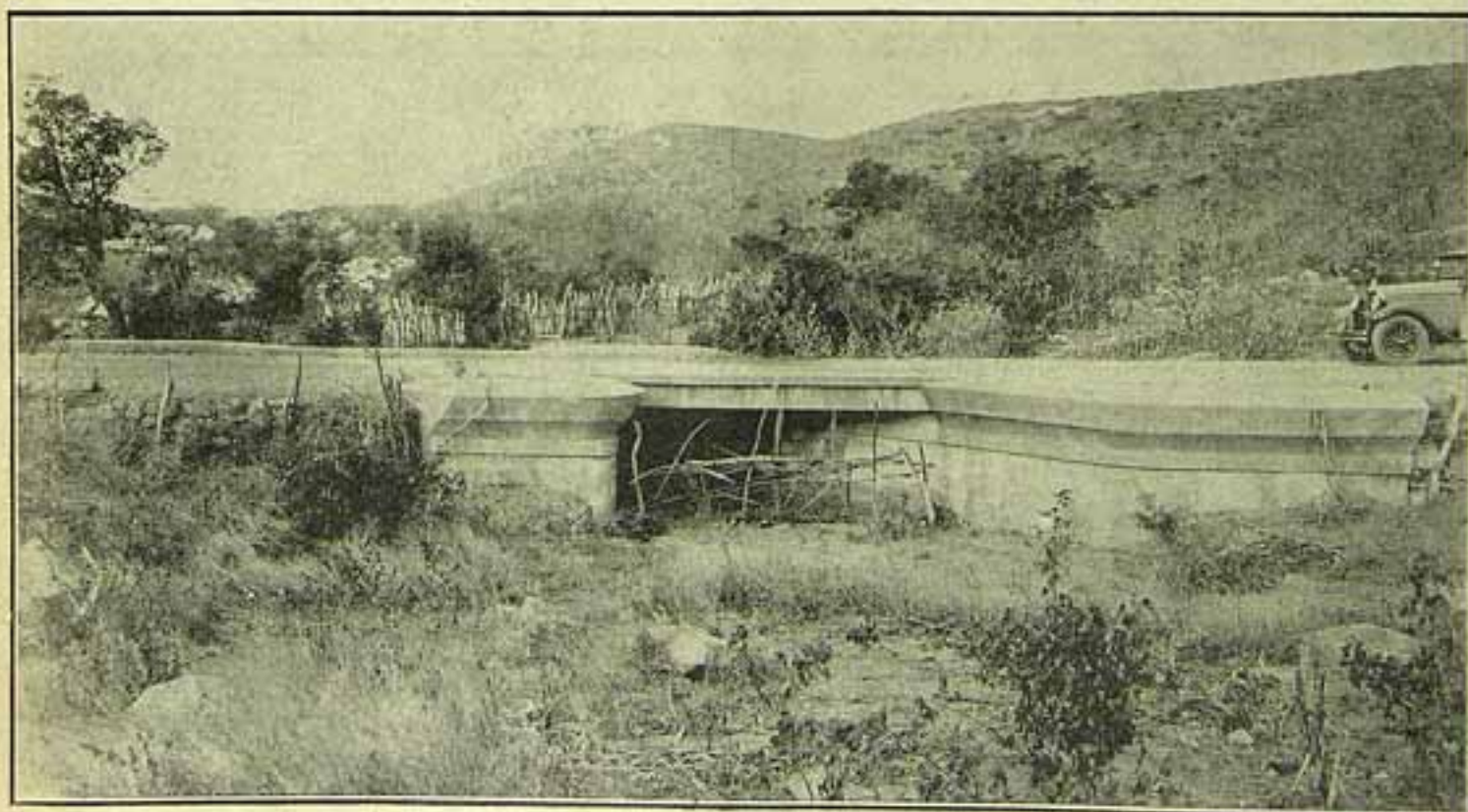
Ramal de Santa Luzia, vendo-se o pontilhão esconso de 3 m. 50 de vão — Kilometro 38
