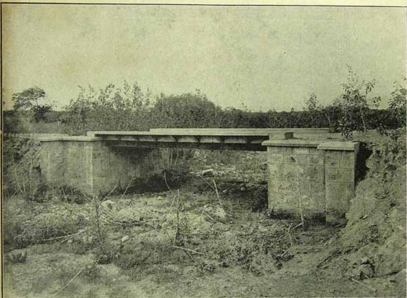
Ponte de 8 metros de vão, na Estrada de Rodagem da Campina Grande a Souza no kilometro 42
