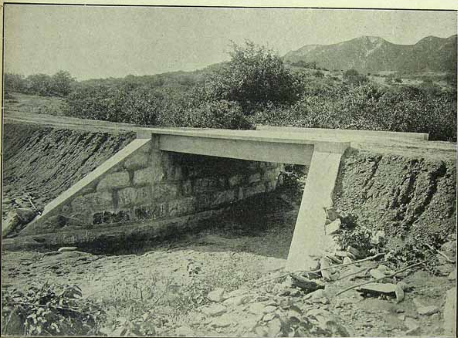
Ponte de 5 metros de vão, na Estrada de Rodagem de Campina Grande a Souza — Kilometro 169
