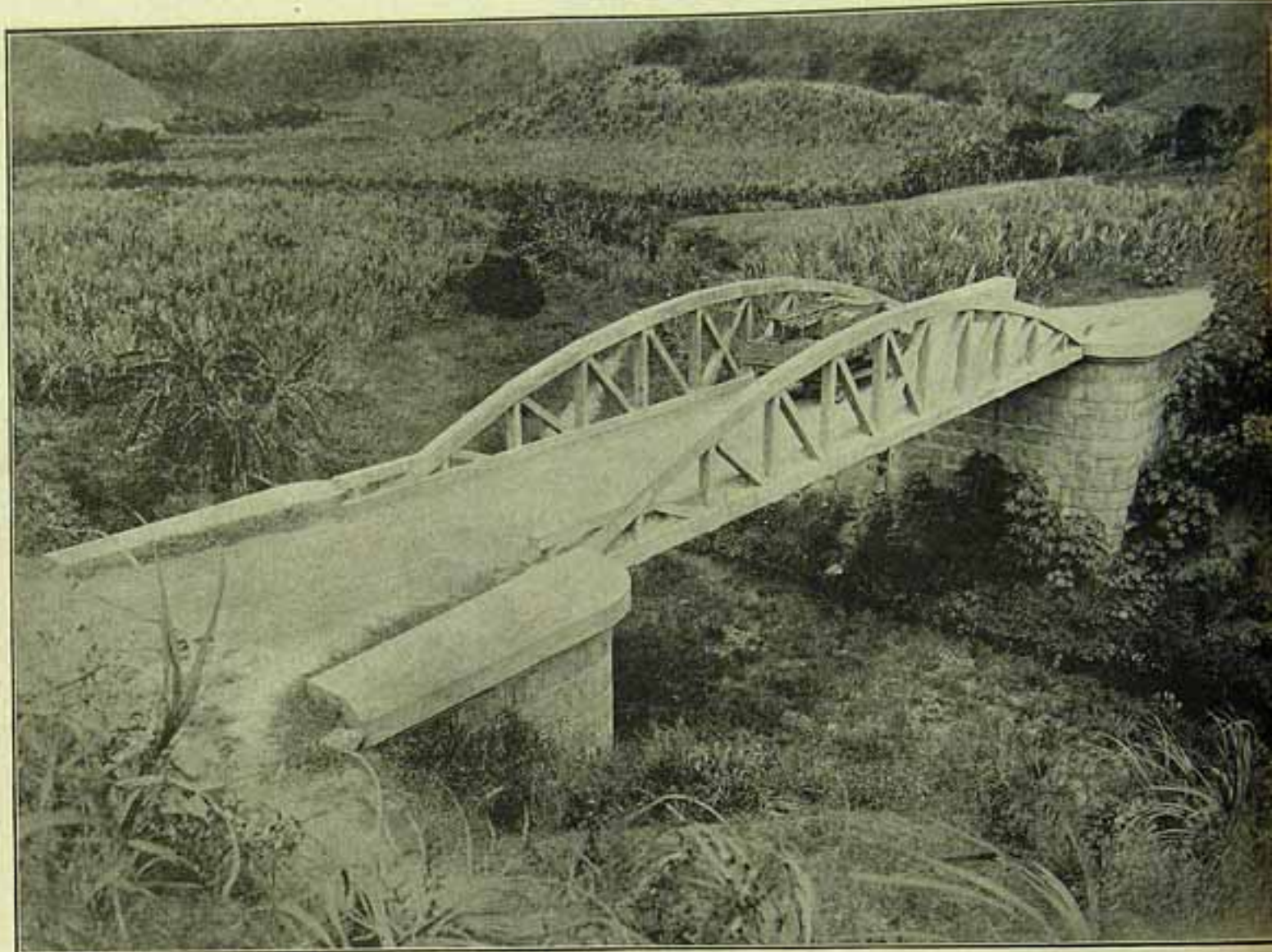
Um encantador aspecto da Estrada de Rodagem Campina Grande-Alagôa Nova, vendo-se a ponte sobre o Rio Urucá
