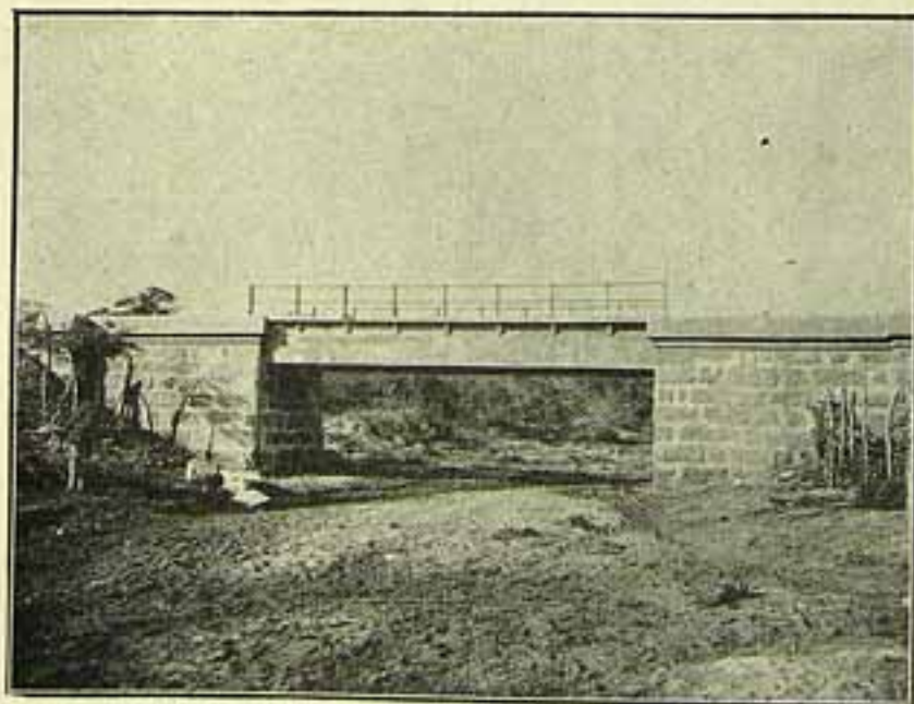
Ponte de 11m.10 de vão na Estrada de Rodagem de Campina Grande a Sousa — Kilometro 20.
