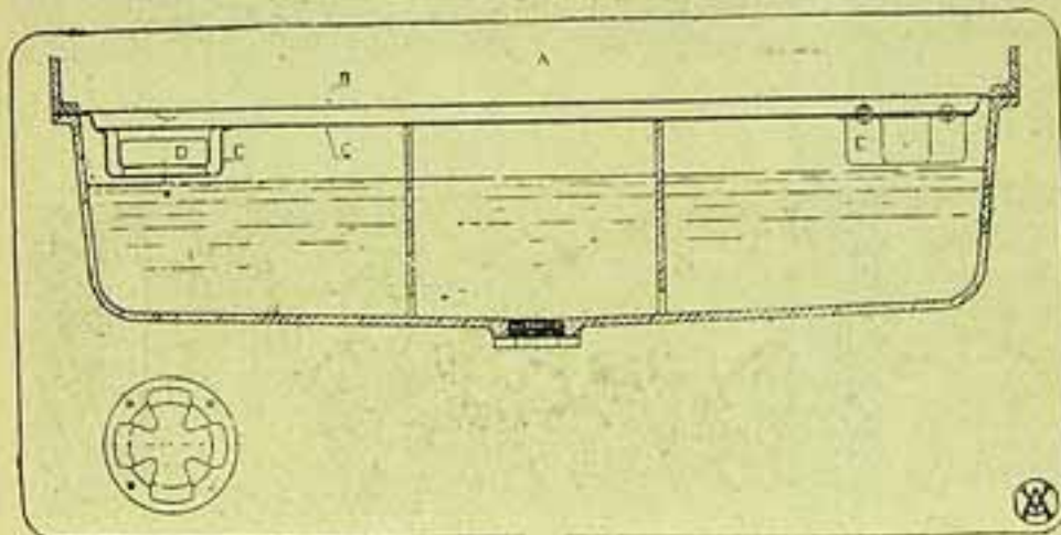
Carter inferior de motor, formando reservatorio de oleo. A folha de ferro C, que o cobre, tem do's orificios em cada extremidade. O lubrificante do motor pode voltar ao carter, mas o oleo do carter não pode invadir o motor; o que é impedido pelos fluctuadores de cortiça D.
