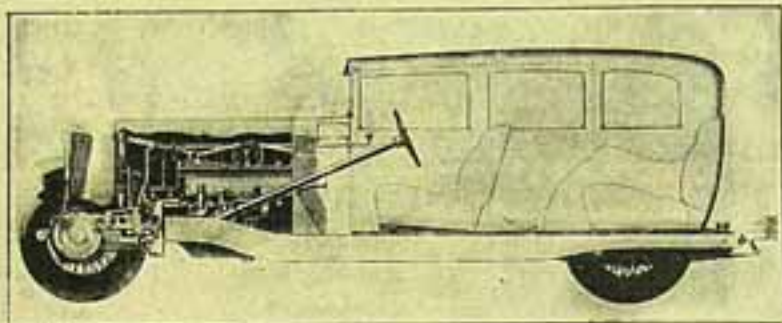
Secção de um Cord, mostrando a armação recta do carro e a planta motriz.
