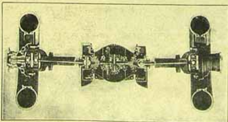
Secção differencial e rodas deanteiras.
