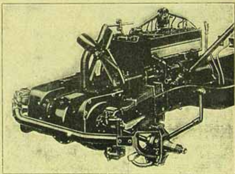
Parte deanteira do motor, mostrando o eixo differencial, transmissão, mola e articulação universal.
