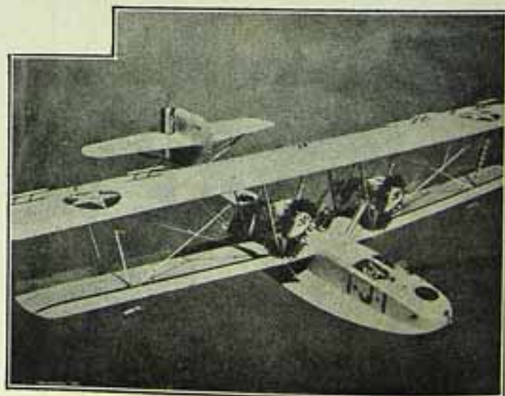
O ultimo modelo de hydro-avião com dois motores voando sobre S. Diego — Argentina.
