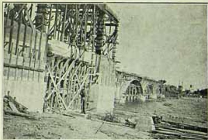
Um dos bate-estacas e a base para o poste fiscal, na margem brasileira
