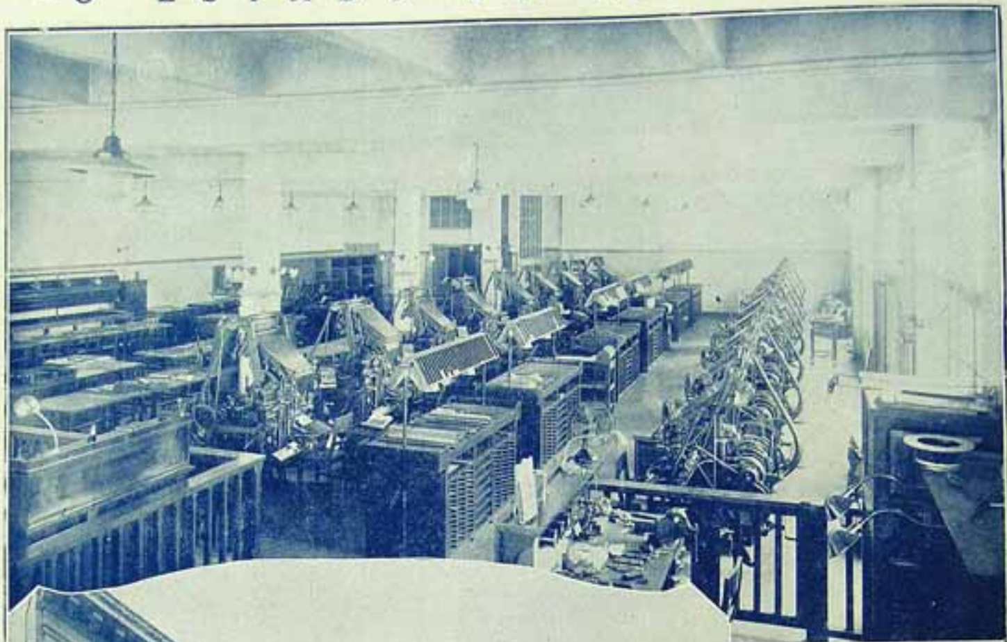
Vista de uma parte dos Linotypes destinada exclusivamente à composição de linha cheia.
