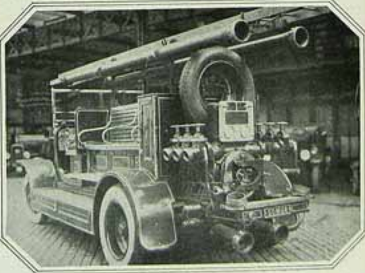
AUTO-BOMBA "SOMUA" — De grande potencia, capaz de alimentar 24 linhas, é utilizada nos grandes sinistros. Descaça — 300 metros cubicos horarios.
