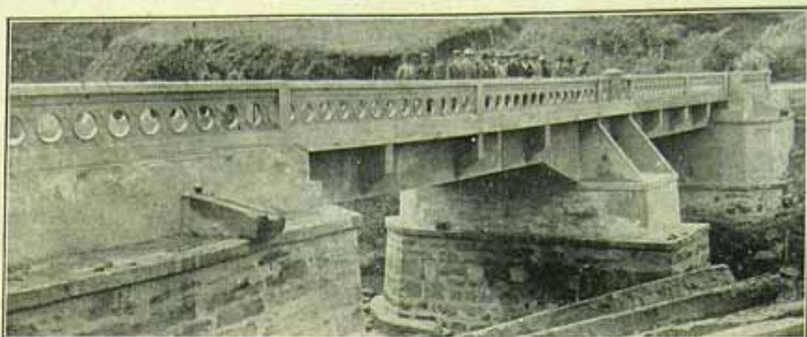
Estrada de Rodagem Belo Horizonte-Rio — O presidente Antonio Carlos visitando a Ponte Zamba, sobre o rio Parahybuna, no trecho de Juiz de Fora a Parahybuna.
