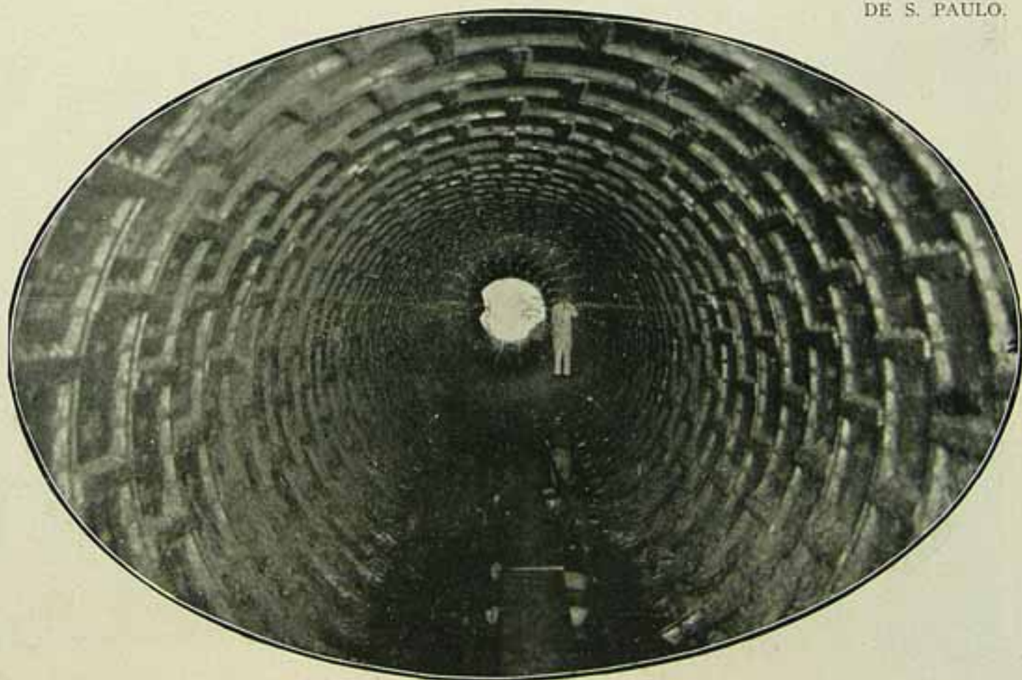
Tunnel em terra, com revestimento de ferro fundido
