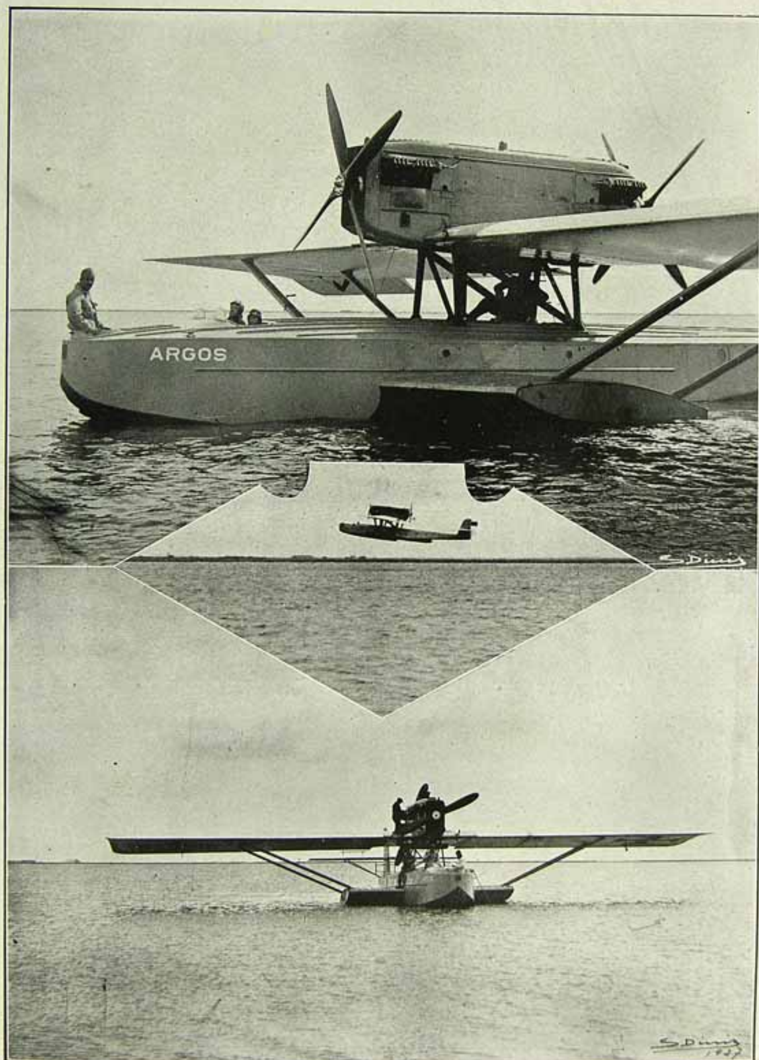
O "Argos" com as hélices de 4 pás, no Tejo, prompto para partir. — No instante supremo: o "Argos" levantando a voo. — O aparelho, horas antes da partida, ainda com as hélices de 2 pás, as quais foram substituídas no ensaio derradeiro.
