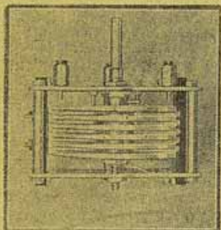
Condensador de variação lineal de frequencia, com laminas em forma de cunha, para produzir o effeito de variação lineal de frequencia.
