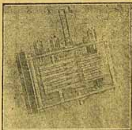
O condensador de variação linear de frequência com as laminas giratorias em posição de maior capacidade, mostrando a reduzida separação destas.
