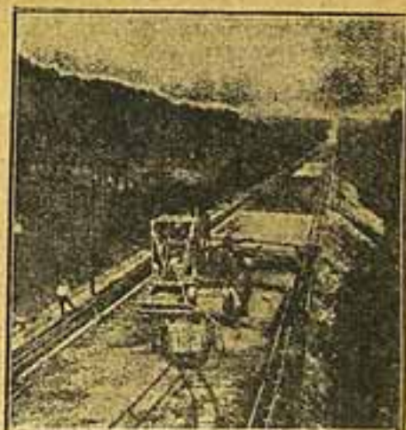
Pavimentação da auto-estrada por meios inteiramente mechnicos e processos modernos
