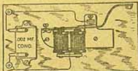
Detalhes do aparelho protector para valvulas
