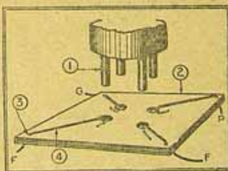
Porta-valvulas rudimentar a que se refere a nota. 1—espigas; 2, papelão grosso; 3, pequenos furos; 4, fio.
