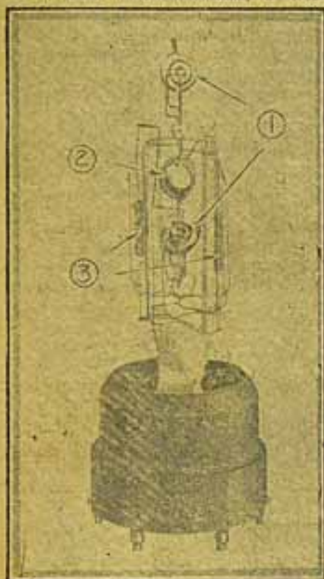
Fig. 5 — O interior da válvula de vácuo na fig. 1. — 1, elementos do amplificador; 2, condensador; 3, resistência.
