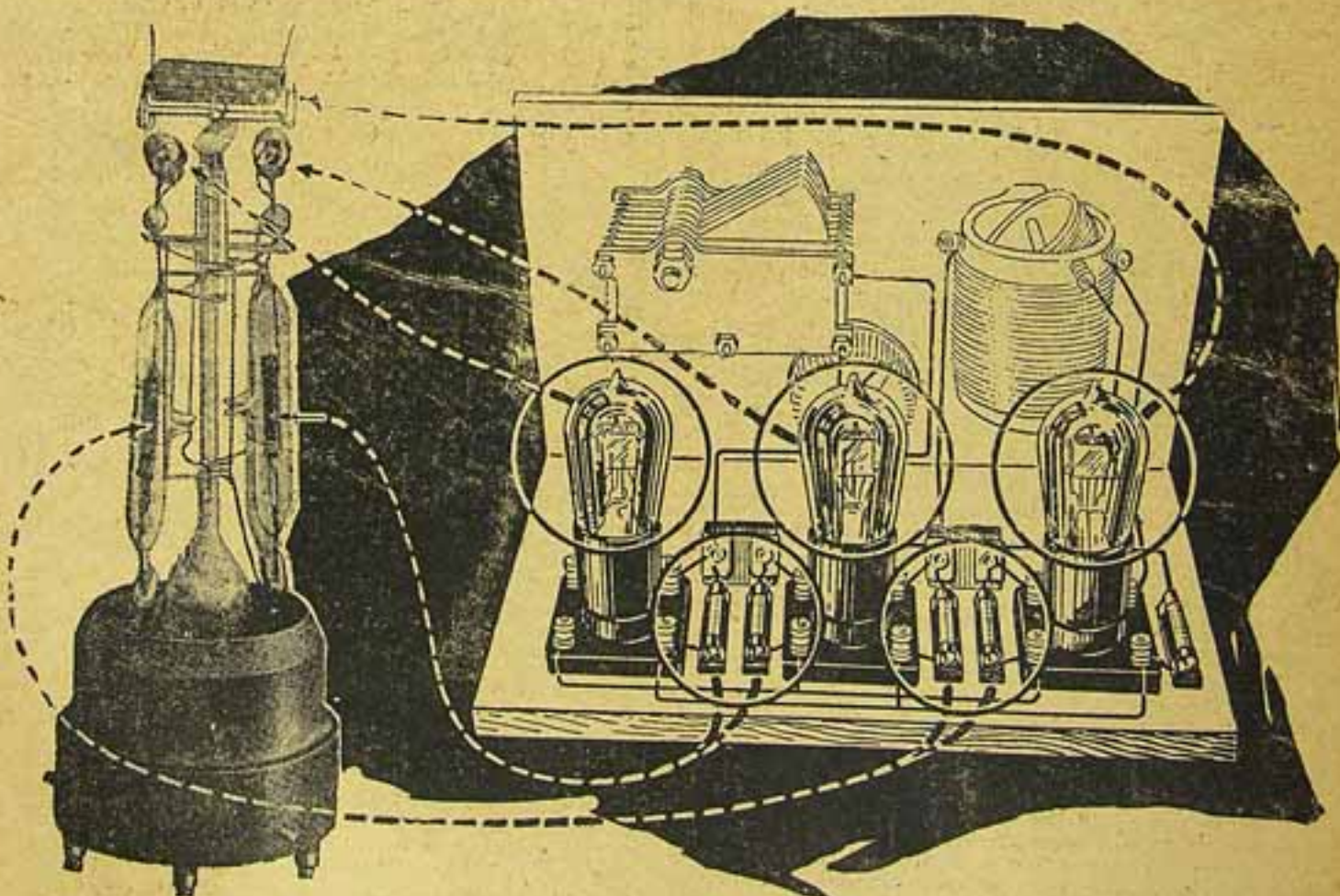
Fig. 5 — Este diagramma representa o numero da válvula e seus apparatus da complexão, que o Dr. Loewe incorpora numa das suas novas válvulas
