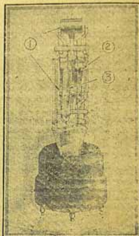
Fig. 3 — Válvula do Dr. Loewe, contendo duas fases de amplificação radio-frequente, de accoplamento mediante resistências. 1, elementos do amplificador; 2, condensador; 3, resistência.
