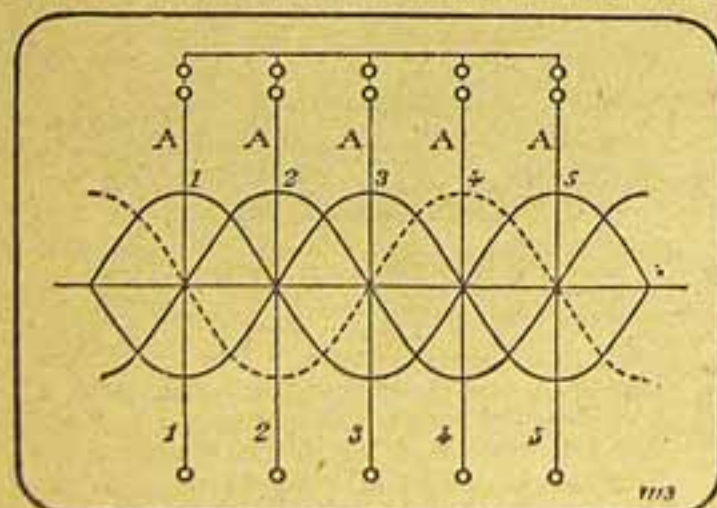
Fig. 6 — Vista da face de um reflector plano do primeiro tipo. — As ondas idênticas emitidas simultaneamente pelas cinco antenas verticaes se destroem mutuamente do plano do reflector.
