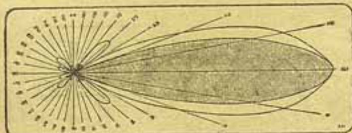
Fig. 9 — Diagramma das intensidades do feixe das ondas dirigidas por um systema reflector comportando 15 antenas em planos verticaes.
