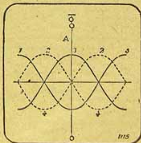
Fig. 8 — Vista de perfil de um reflector plano de segundo tipo. — As ondas emitidas simultaneamente pelas cinco antenas são cada uma em phazas differentes que correspondem aos afastamentos reciprocos das antenas, se ajustam na direcção do reflector e se annullam umas às outras na direcção perpendicular.
