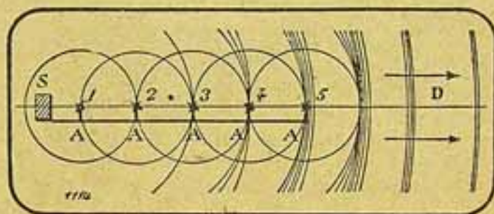
Fig. 7 — Emissão de um feixe de ondas dirigidas por um reflector plano de segundo tipo. — 1, 2, 3, 4, 5, p te das antenas verticaes; A, S, estação de emissão ligada às antenas por linhas cujos comprimentos differem entre si um quarto de onda; D, direcção do feixe das ondas reflectidas, parallelas ao plano do espelho.
