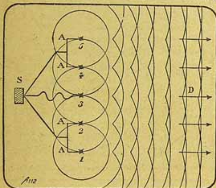
Fig. 5 — Emissão de um feixe de ondas dirigidas por um reflector plano do primeiro tipo. — 1, 2, 3, 4, 5, p te das antenas verticaes; S, estação de emissão ligada às antenas por linhas de igual comprimento; D, direcção do feixe das ondas. Ondas reflectidas.
