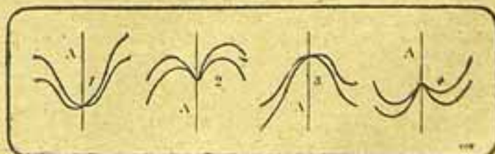
Fig. 4 — Partida das ondas irradiadas por diversas antenas verticaes elementares em duas direcções perpendiculares. A, Antenas elementares verticaes; 1, ondas no minimo de amplitude; 3, ondas no maximo de amplitude; 2 e 4, ondas partindo em duas posições intermediarias das precedentes.
