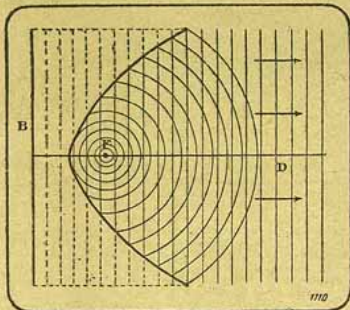
Fig. 3 — Reflexo da irradiação das ondas sobre um cylindro parabolico. — F, emissor situado no foco; B, directriz da parabola, donde parece provir o feixe das ondas reflectidas.
