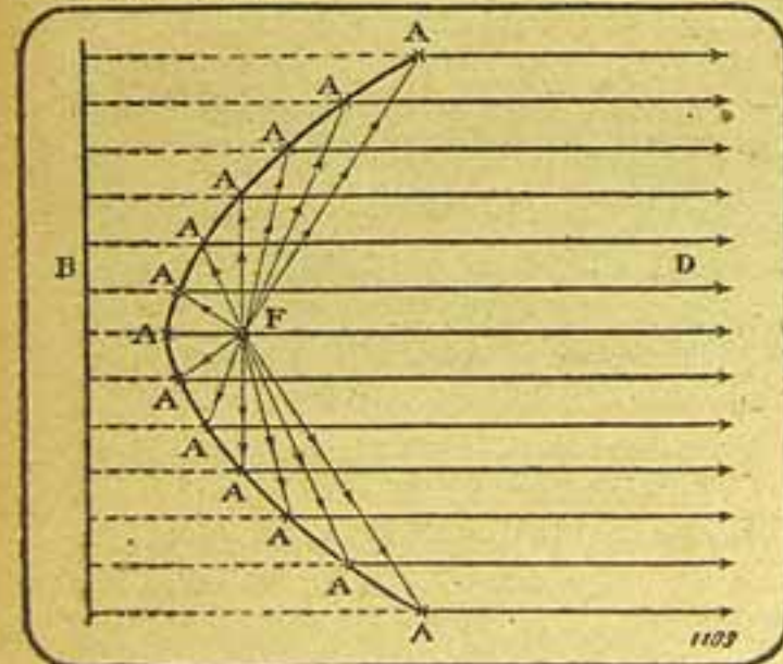
Fig. 2 — Reflexo da direcção das ondas sobre um cylindro parabolico. A, pt. das antenas verticaes; P, emissor situado no foco; B, directriz da parabola, donde parece provir o feixe das ondas reflectidas na direcção D do eixo de espelho.
