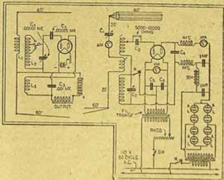
Fig. 1 — Esta gravura mostra o circuito Meissner para transmittir ondas de 40 a 80 metros de comprimento. Este transmissor emprega a corrente da iluminação electrica.
