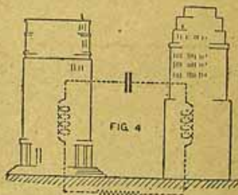
O esqueleto do aereo, os encanamentos, etc., existentes nos edificios e entre elles podem formar um systema oscillatorio, como demonstra a illustração.
