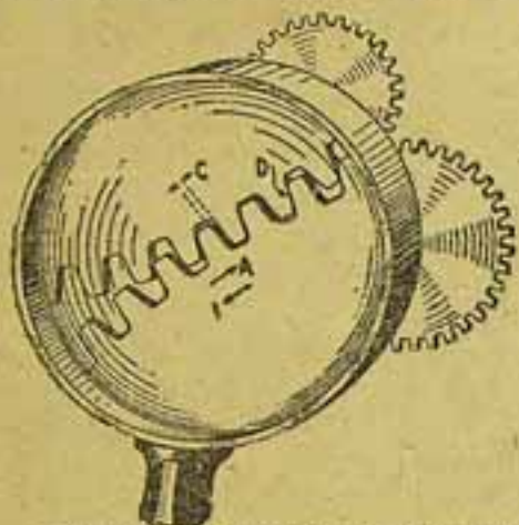
Figura 5. — Na direcção de A não há "jogo" algum, devido a que as engrenagens formam contacto em D. Si invertermos o movimento teremos de eliminar o espaço em C.
