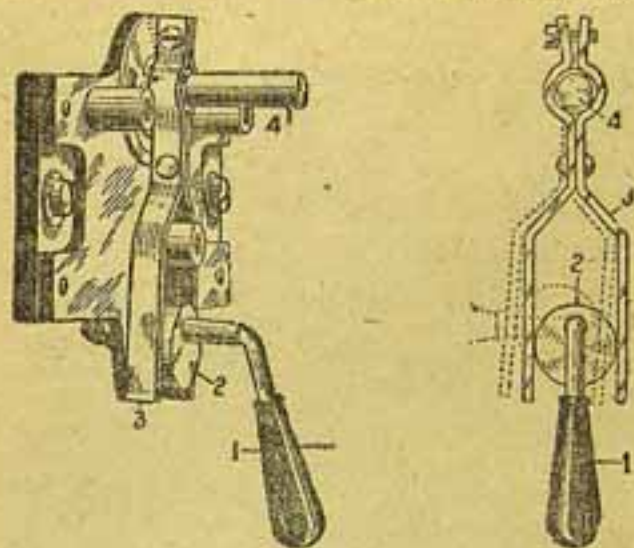
Figura 4. — Um tipo de movimento de redução muito conhecido. Ao mover-se a excentrica (2), move-se o eixo (3), o qual faz girar o eixo do condensador (4) por meio do collar que o suporta.
