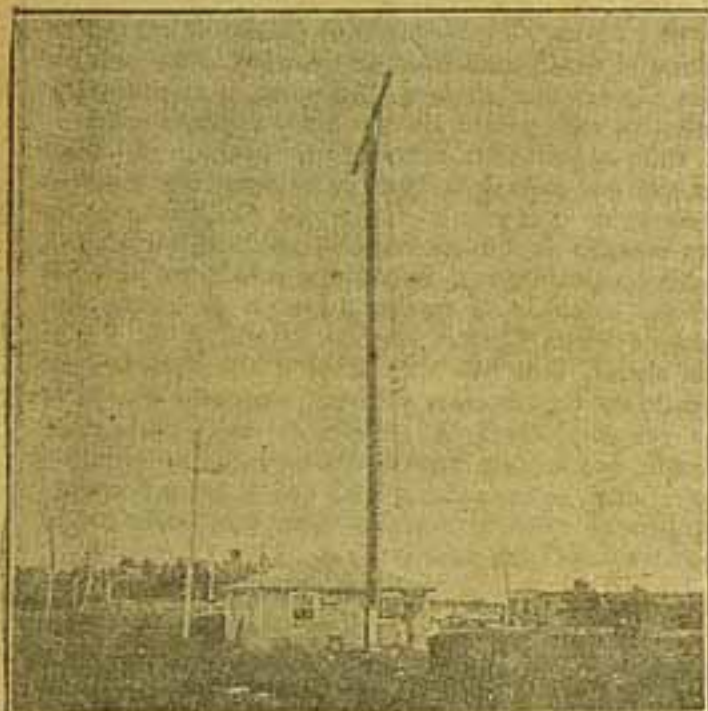
A parte vertical da antenna que constitue o factor mais importante na geração das ondas polarizadas. Em cada uma das secções verticaes da antenna deve existir equilibrio absoluto da corrente para poder obter resultados maximos.
