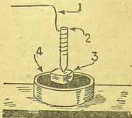
Fig. 5 — Um pedaço de barra de lapis bem espontado ou de antimonio forma um contacto excelente para se empregar com galena ou silico. 1, contacto; 2, barra de lapis; 3, crystal; 4, "taça".
