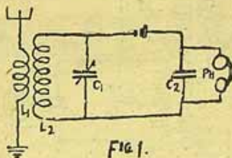
Fig. 1 - Circuito de uma das formas mais simples de receptores de crystal com accoplamento indutivo.
