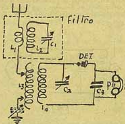
Fig. 2 — Um receptor de crystal pôde tornar-se mais selectivo si se lhe ajunta um filtro da maneira aqui demonstrada.
