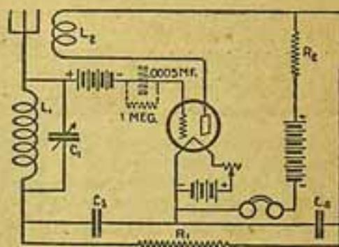
Um dos circuitos "super" mais facéis de construir. Este circuito é muito simples e de fácil manejo.
