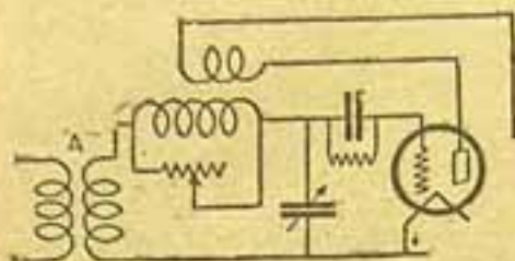
Fig. 1 — Este diagramma reproduz o circuito básico no qual se funda o funcionamento do receptor. Este circuito é muito parecido com o circuito corrente de syntonizador triplo, mas seus resultados são muito melhores.
