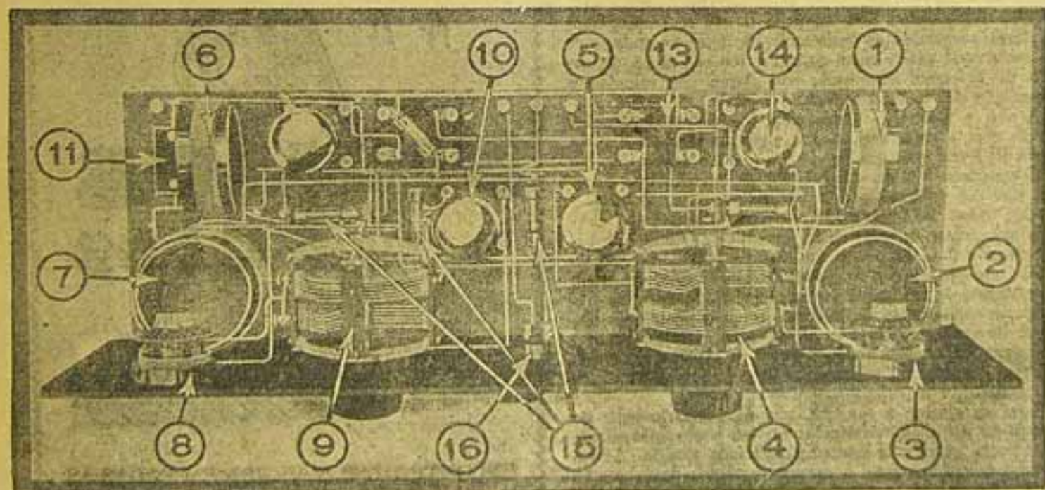
Vista de plano do autor-regenerador. 1 — Bobina de accoplamento de antenna. 2 — inductancia do secundário e bobina de reacção da valvula de radiofrequencia. 3 — Alta resistencia do estagio de radiofrequencia. 4 — Condensador de syntonía de radiofrequencia; 5 — Valvula de radiofrequencia. 6 — Bobina de accoplamento inter-valvular. 7 — Inductancia de carga do secundário do detector; 8 — Alta resistencia do circuito do detector. 9 — Condensador de syntonía do detector. 10 — Valvula detectora. 11 e 13 — Transformadoras de audiofrequencia. 12 e 14 — Valvulas de audiofrequencia. 15 — Resistencia "Amperite". 16 — Commutador do filamento.
