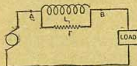
Fig. 2 — Do principio sobre o qual se baseia o circuito da fig. 1, deriva-se o phenomeno que ocorre com esta diagramma de connexão. As resistencias A e B variam o necessario para regular automaticamente as oscillações espontaneas.
