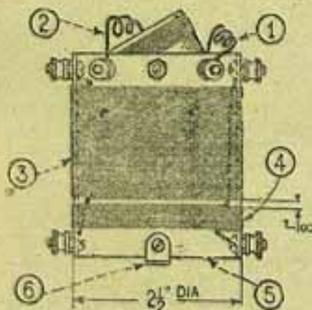
Fig. 3 — Conexões flexíveis do rotor; 3 — Abolínado do secundario (60 voltas de fio n. 24 com revestimento duplo de algodão); 4 — Primario (10 voltas, idem, idem); 5 — Tubo de papelão; 6 — Supporte para montar o accoplador variavel.
