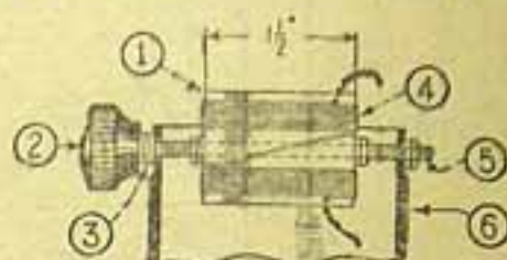
Fig. 4 — 1 tubo de papelão; 2 — Frente; 3 — Arruelas separadoras; 4 — Rotor (30 voltas de fio n. 26 com revestimento duplo de algodão); 5 — Barra com roza de 3 1/2 pollegadas; 6 — Parte posterior.
