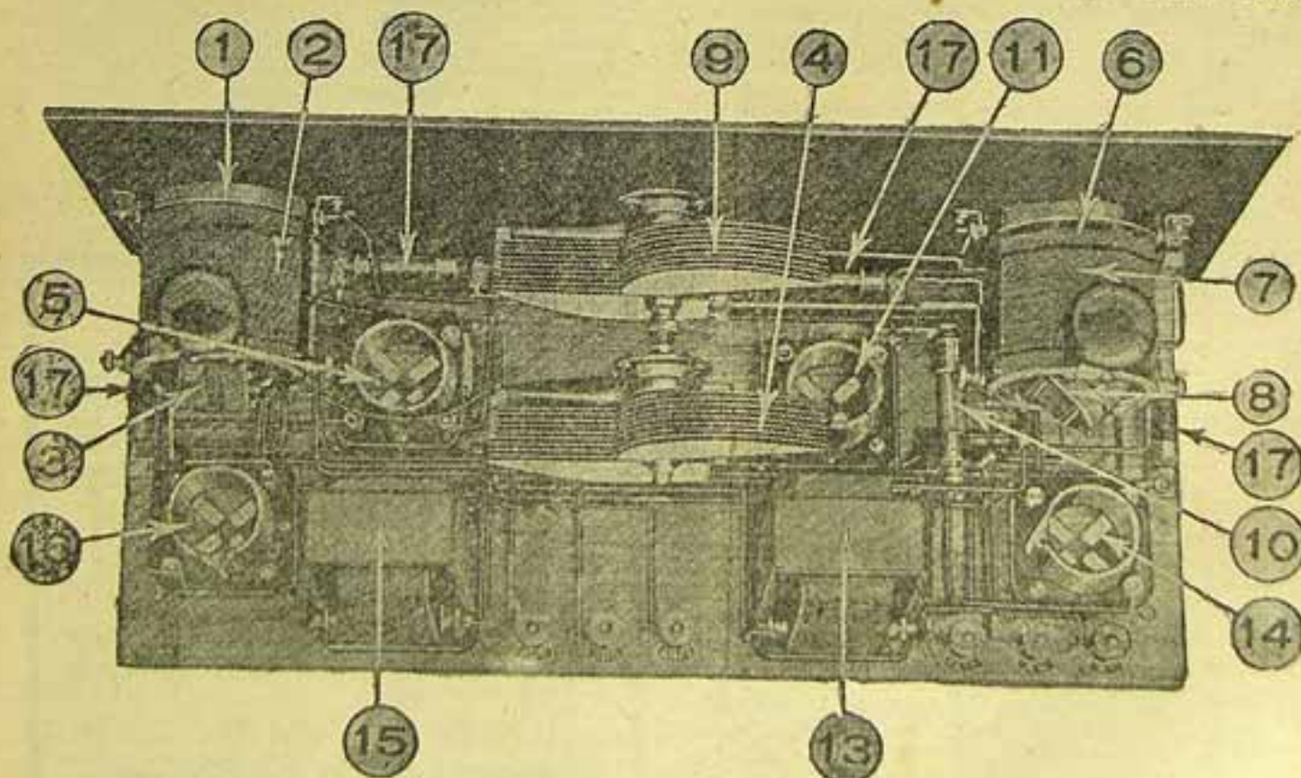
Vista superior do novo circuito indicando a disposição das diferentes partes. Todos os numeros de todas as illustrações correspondem entre si. Note-se a conexão que une as condensadores variáveis (4) e (9) e a maneira adequada em que vão collocadas todas as partes que compõem este receptor.
