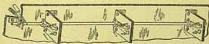
Fig. 4 — Schema da fig. 3. Aqui não são vistos os condensadores fixos, mas sim a construção dos comutadores de mudança.
