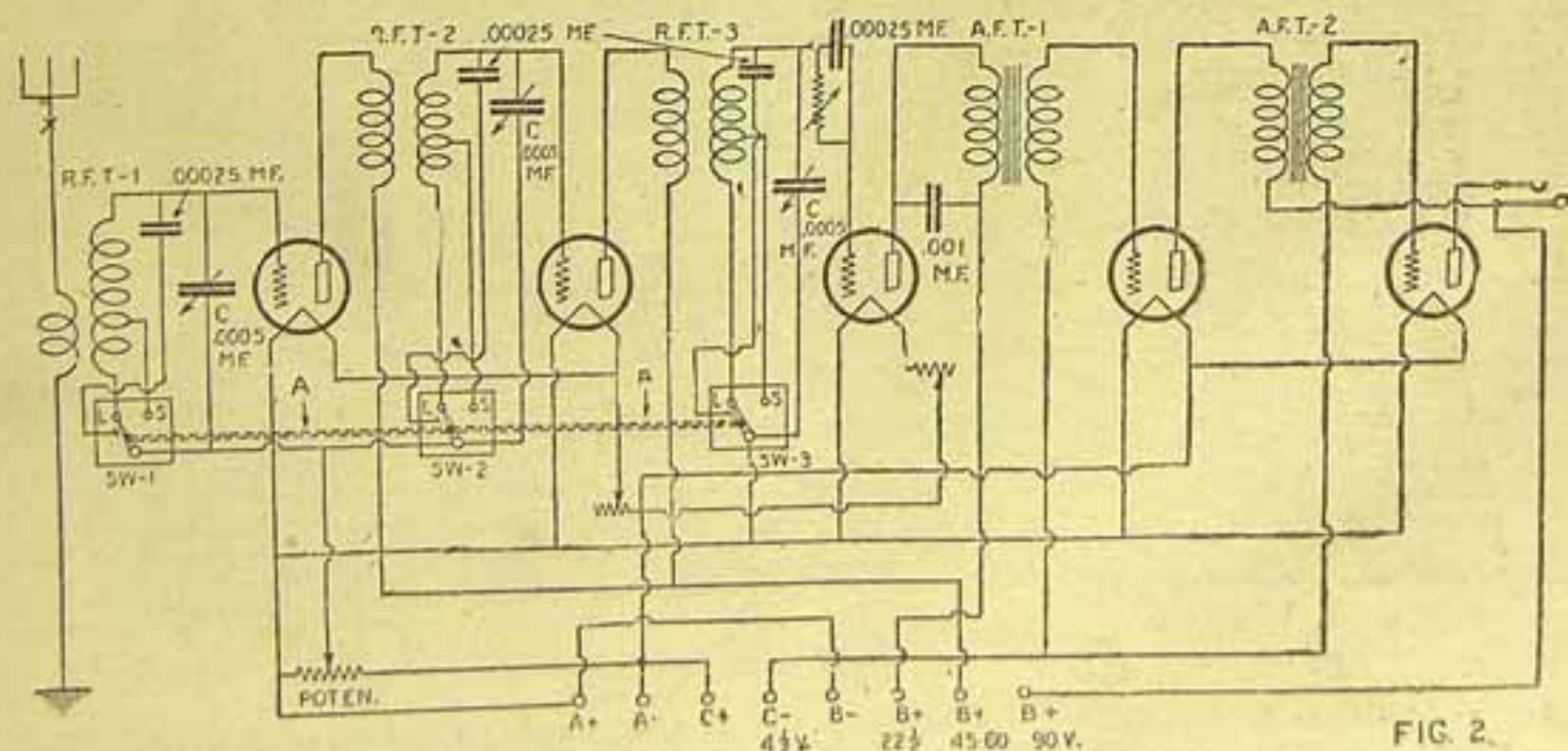
Fig. 2 — Diagramma do circuito do receptor. Os tres commutadores são manejados por meio do eixo marcado com a linha pontuada. Note-se especialmente a ligação dos condensadores fixos em cada passagem de syntonia.
