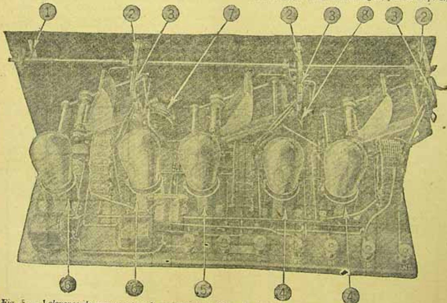
Fig. 5 — 1, alavanca do comutador; 3, condensadores fixos de 0.00025 mfd.; 4, amplificadores de radio frequência; 5, detector; 6, amplificadores de audio-frequência; 7, reostato; 8, potencímetro; empregam-se condensadores variaveis, de variação lineal. Note-se a vareta de materia isolante que acciona os tres comutadores simultaneamente.
