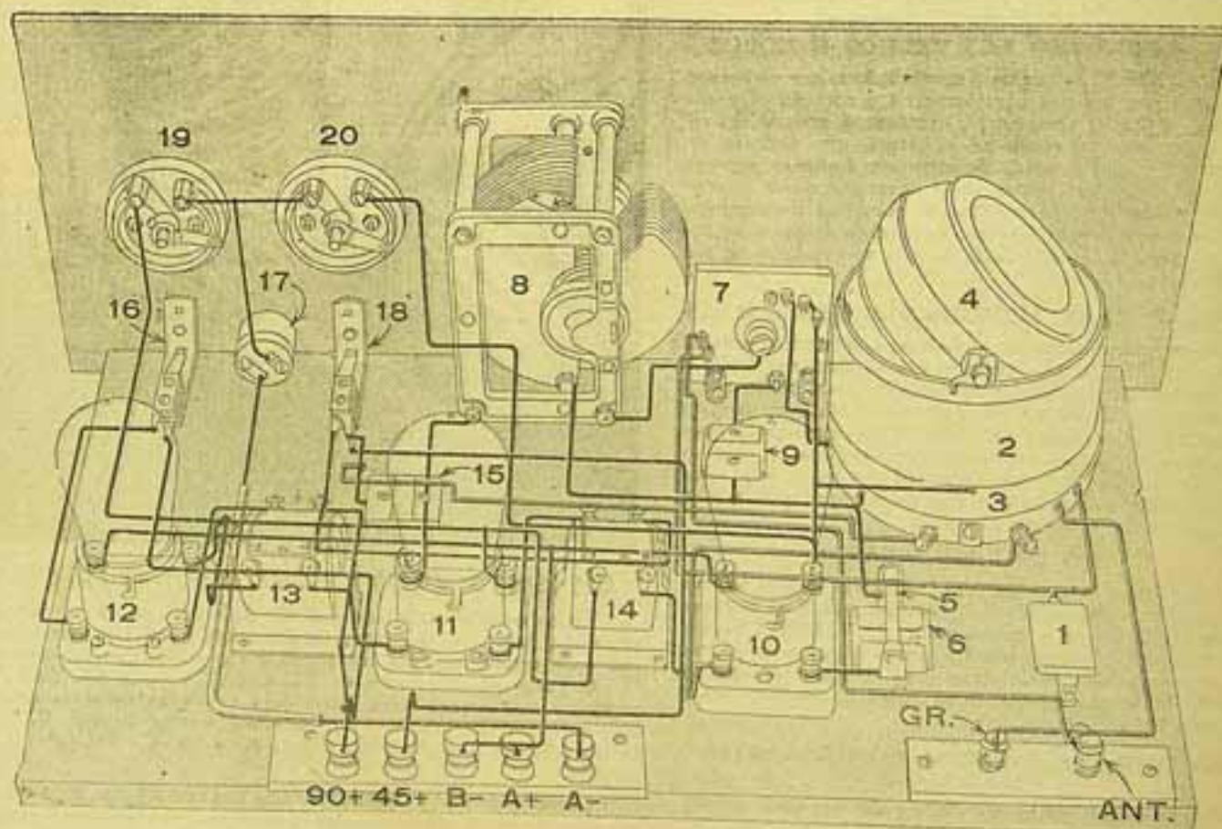
Fig. 4. — Disposição das diferentes partes no receptor. 1, Condensador; 2, bobina secundaria; 3, bobina primaria; 4, bobina de reacção; 5, resistencia de escapamento; 6, condensador de regagem; 7, commutador especial; 8, condensador variavel de 0,0005 mfd's; 9, condensador fixo de 0,0005 mfd's, connectado em parallelo com o condensador de baixa frequencia; 10, valvula detectora; 11 e 12, valvulas amplificadoras; 13 e 14, transformadores de circuito duplo; 15, condensador de estagio; 16, ajustamento das valvulas simplificadoras e 20, rheostato da valvula detectora.
