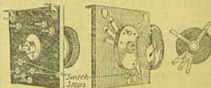
Fig. 2. — Os contactos do commutador podem ser feitos muito facilmente.
