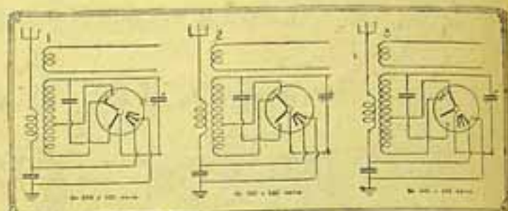
Fig. 3. — Esses diagrammas mostram o commutador em tres posições diferentes. O alcance é approximadamente: 1.ª posição, de 600 a 400 metros; 2.ª posição, de 420 a 220; 3.ª posição, de 240 a 140 metros.
