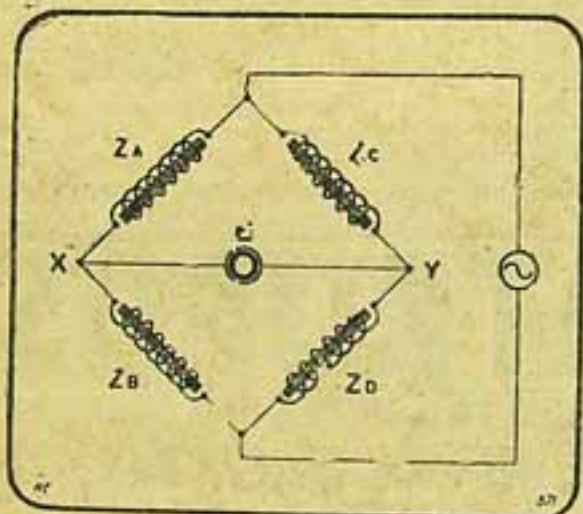
Fig. 1 — Schema de montagem para a experimentação dos enrolamentos dos transformadores por um methodo de zero em alternativa.
