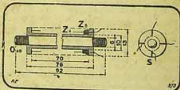
Fig. 3 — Realisacão das bobinas exploradoras. — As cotas são indicadas em millimetros. A bobina é fraccionada.
