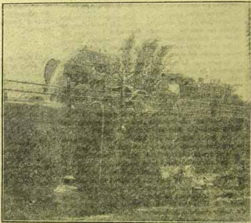
Automovel irrigador, construido pelos irmãos Barbosa, de S. Carlos, especialmente para os serviços de estradas. Possui um dispositivo privilegiado pelo qual apanha a agua em qualquer ponto da estrada, elevando-a a mais de 6 metros, como mostra a photographia.
