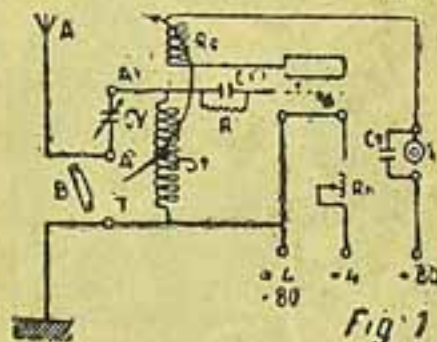
Fig. 1 — Schema de principio
