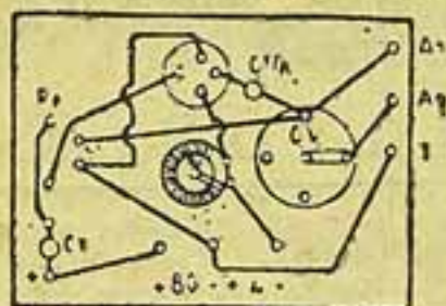
Fig. 2 — Plano de montagem
