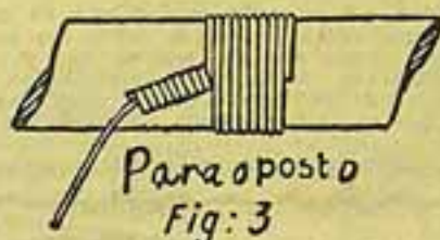
Connexões do fio de tomada de terra
