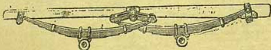
Novo tipo de molas "Rickenbacker", que constitui uma das últimas novidades do automobilismo: mola dupla, construída com o intuito de absorver choques horizontais.
