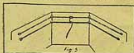
Fig. 5. — Antenna em U
