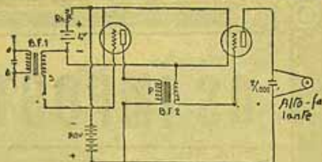
Fig. 2. — Schéma de montagem do alto-falante
