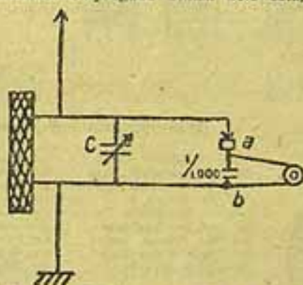
Fig. 1. — Schéma do posto de galena
