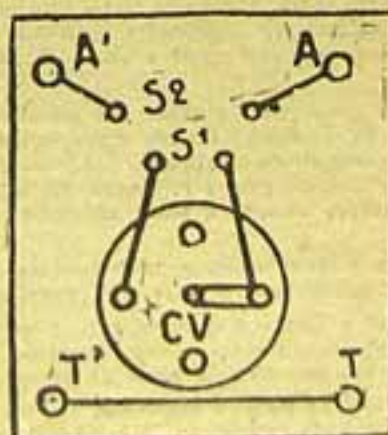
Fig. 4. — Montagem em Tesla
