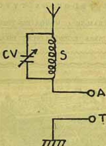
Fig. 1. — Circuito filtro directo
