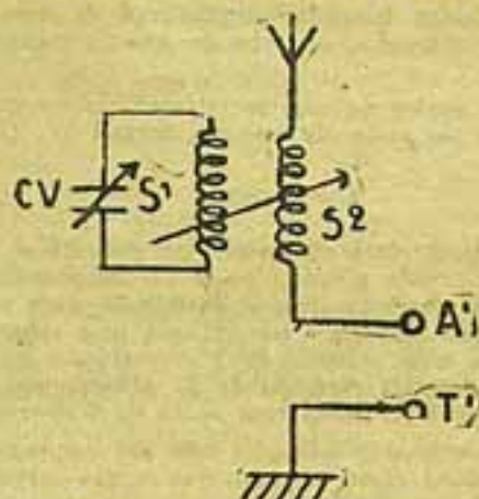
Fig. 2. — Circuito filtro Tesla
