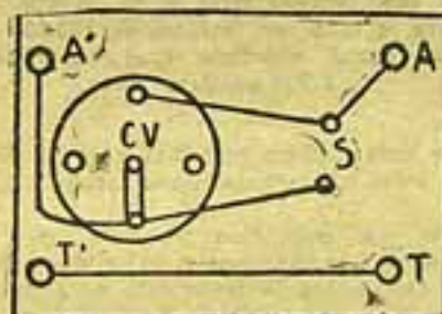
Fig. 3. — Montagem em directo
