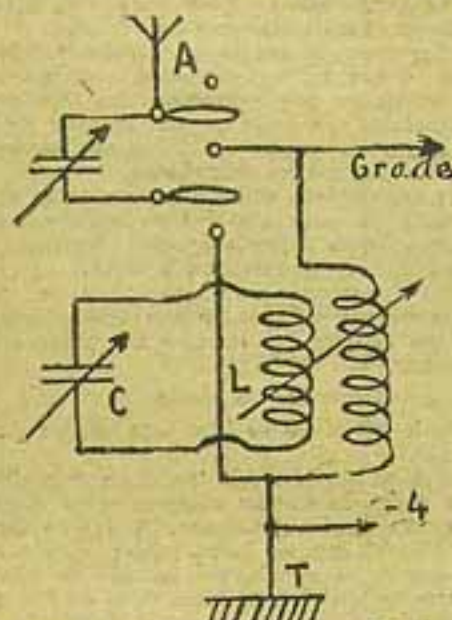
Fig. 2 — Filtro de absorpção simples. C. L. circuito de accórdo filtrador ou ondometro
