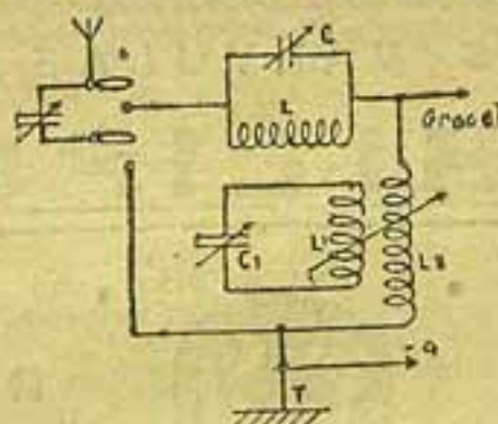
Fig. 3 — Filtro de absorpção duplo C. L. circuito de blocagem; L. C. circuito de absorpção
