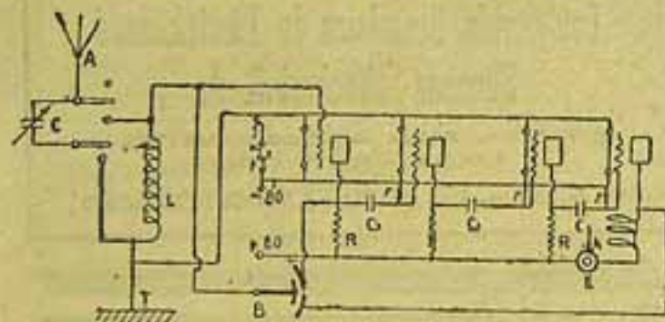
Fig. 1 — O amplificador classico de resistencias; C — 1:1.000; L — ninho de abelha ou bobina cylindrica de cursor; R — 80.000 ohms; r — 2 megohms; c — 20/100.000; K — 200 espira 3/10 de 8 centímetros diametro em vrac; B — compensador de "accrochagem" comportando uma lamina movel entre duas laminas fixas
