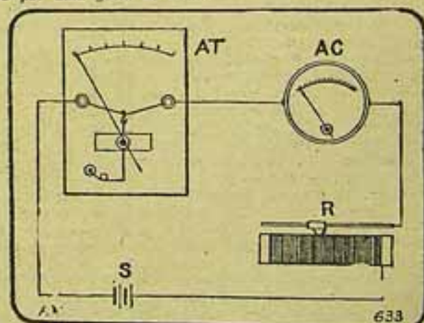
Fig. 3 — AFERIÇÃO DO AMPEREMETRO DE ANTENNA. — AT, amperemetro de antenna; AC, amperemetro de corrente continua, ligado em série; S, bateria de acumuladores de aquecimento; R, reostato.
