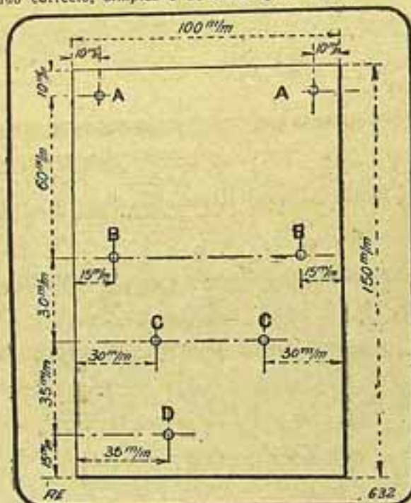
Fig. 1 — PLAQUETTE DE EBONITE FURADA TRAZENDO O AMPEREMETRO DE ANTENNA. — AA, furos de fixação da graduação; BB, furos de fixação do fio thermico; CC, furos de fixação do eixo da agulha indicadora; D, furo de fixação da mola de reversão.
