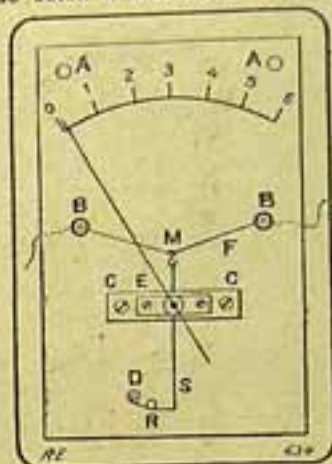
Fig. 2 — MONTAGEM DO AMPEREMETRO DE ANTENNA. — AA, parafusos do quadrante; BB, bornes do fio aquecido; CC, suporte do "pivot" da agulha E; R, mola fixada em D; F, fio aquecido; M, gancho fixando o fio que dirige a agulha.
