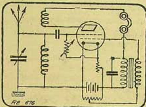
Fig. 4 — MONTAGEM REFLEXA SEM BATERIA DE PLACA, UTILIZANDO UMA LAMPADA DE DUAS GRADES. — Emprego de um transformador de baixa frequencia, cujo primario é shuntado por um condensador; emprego de um potenciometro de grade e da reacção
