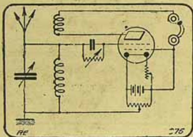
Fig. 3 — MONTAGEM SEM BATERIA DE PLACA UTILIZANDO UMA LAMPADA DE DUAS GRADES. — Emprego de um potenciometro de grade e da reacção. Detecção por condensador shuntado variavel
