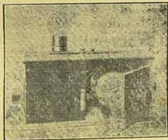
Fig. 5 — RECEPTOR REFLEXO SEM BATERIA DE PLACA. — C, condensador variavel; A e T, bornes, antena e terra; E, bornes do phone; F, bornes da bateria de aquecimento; B1, B2, bobina em ninho de abelha; R, rheostato de aquecimento; P, barrette de recorte para se introduzir a bateria eventual de placa
