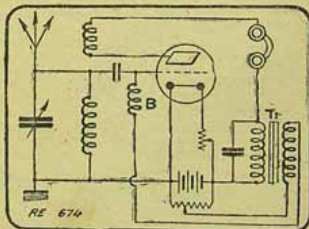
Fig. 2 — CIRCUITO "REFLEXO" COWPER FUNCIONANDO SEM BATERIA DE PLACA. — B, bobina de choque evitando a derivação para a terra das oscillações de alta frequencia; Tr, transformador de baixa frequencia com primario shuntado. Emprego dum potenciometro
