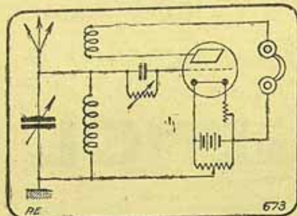
Fig. 1 — MONTAGEM SEM BATERIA DE PLACA DO EXERCITO BRITANNICO (1918). — A placa é ligada por intermédio da bobina de reacção e do telephone ao polo positivo da bateria de aquecimento de 6 volts; o rheostato está na extremidade positiva do filamento. Potenciometro de 300 ohms regulando a tensão media da grade e reacção
