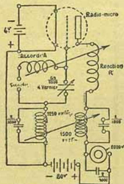
Schema de montagem
