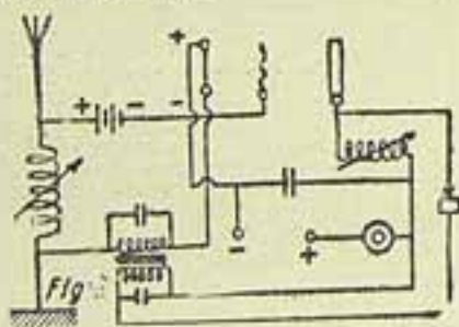
Fig. 2 — Montagem com pilha
