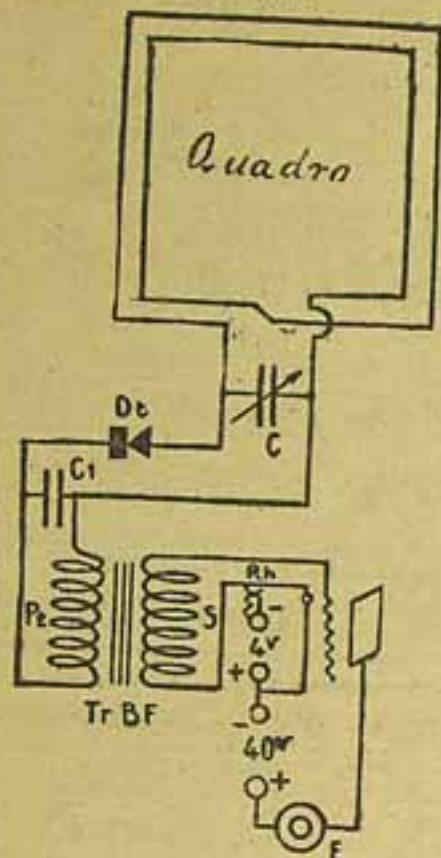
Fig. 1 — Schema da montagem
