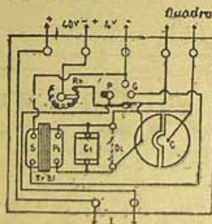
Fig. 2 — As ligações internas
