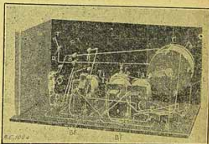
Fig. 3 — Montagem do novo amplificador de baixa frequência — T, borne terra; C, condensador variavel; P, S, R, supports das bobinas do primario, secundario e reacção; Q, condensador shuntado; D, BF, supports das valvulas resistencia 5; K, condensador fixo de 0,001 micropharadi; detectoras e amplificadoras; T1, T2, T3, transformadores de E, bornes da escuta ou bornes do auto falante
