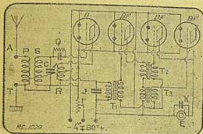
Fig. 1 — Schema do novo amplificador de baixa frequência — A, antena; T, terra; P, bobina primária; S, bobina secundária; R, reacção; C, condensador de accordo; Q, condensador shuntado; I, condensador fixo, de 0,001 micropharadi; r, rheostato de aquecimento; T1, T2, T3, transformadores de resistencia; K, condensador de 0,002 micropharadi; E, escuta ou auto falante; D, detectora; BF, valvulas amplificadoras de baixa frequência. Pode-se empregar valvulas radio micro
