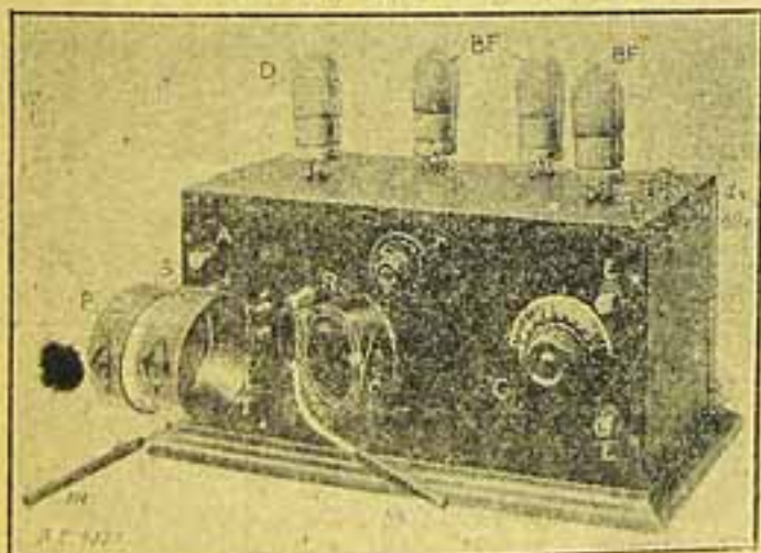
Fig. 2 — Novo amplificador de baixa frequência. — D, detectora; BF, valvulas de baixa frequência; A, borne da antena; P, borne terra; P, S, bobinas primario, secundaria e reacção; r, rheostato de aquecimento; C, condensador variavel; E, bornes da escuta; m, manetas de manobra das bobinas
