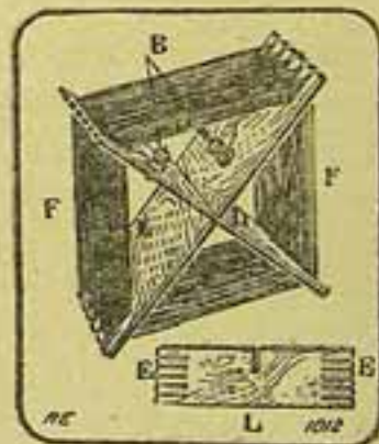
Nova bobina com separação interior — F, bobinagem de fio com uma camada nas fendas das travessas de madeira; B, bornos da extremidade; L, reguas finas de madeira; E, fendas praticadas nas reguas
