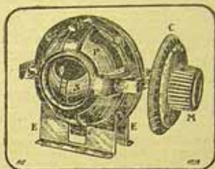
Novo tipo de variometro — C, disco graduado; M, maneta de regulagem; E, esquadros de fixação; P, circuito primario sem apoio; S, circuito secundario sem apoio
