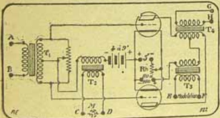
(Fig. 4) — MONTAGEM PUSH-PULL DESTINADA A USOS MULTIPLOS. — A, B, circuito de entrada após detecção; T1, transformador a tomadas symetricas; M, microphone; T2, transformador microphonico; Rh, rheostato de aquecimento; T3, transformador de modulação; T4, transformador de amplificação para o controle
