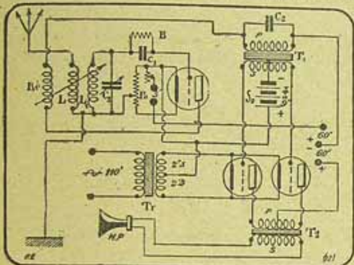
(Fig. 3) — LAMPADA ELECTRICA DE REACÇÃO SEGUIDA DE UM ESTAGIO DE AMPLIAÇÃO A BAIXA FREQUENCIA EM PUSH-PULL, COM AQUECIMENTO EM CORRENTE ALTERNATIVA. — L, L1, variômetros; Ré reacção; C1, C2 condensadores de detecção e de accordo; Pc potenciometro; Tr transformador de alimentação do filamento; T1, T2, transformadores push-pull; HP, alto-falante
